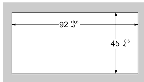
Schalttafel Ausschnitt gemäß DIN 43700-96x48mm
